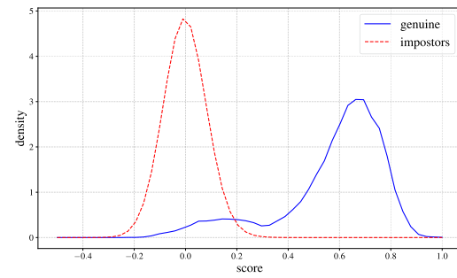
(b) BFW
